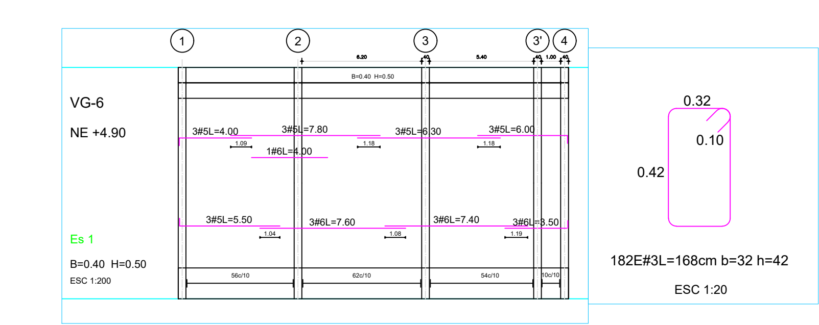
DESPIECE VIGAS DE CUBIERTA –MODULO ESTRUCTURAL 1–
